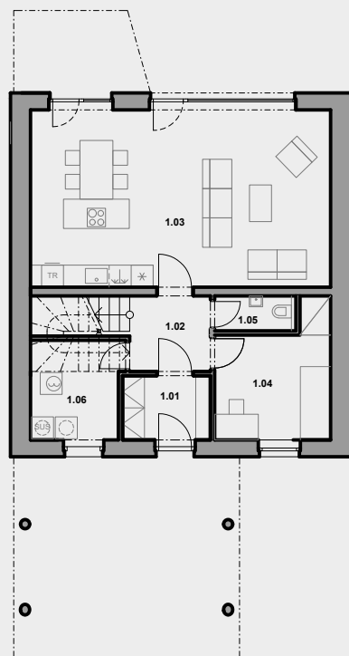
PŮDORYS 1.NP
