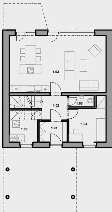
PŮDORYS 1.NP
