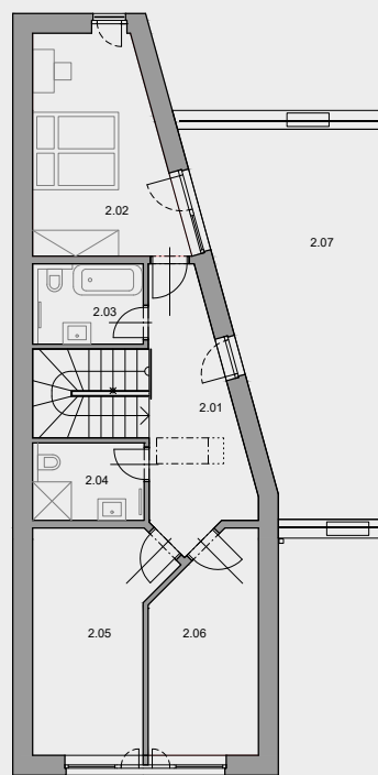
PŮDORYS 2.NP
