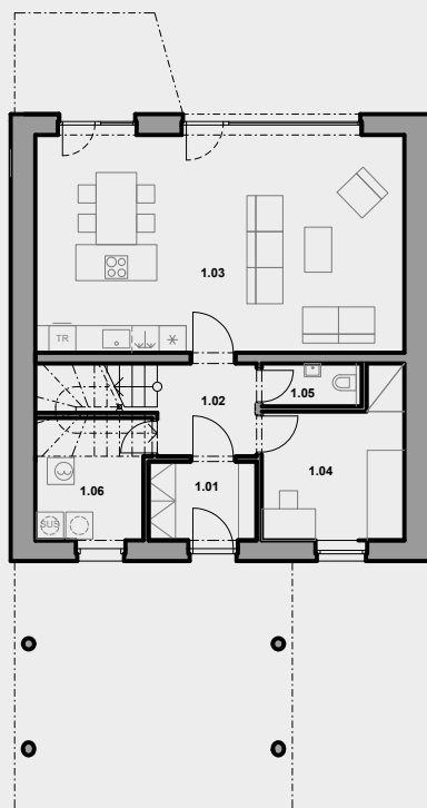
PŮDORYS 1.NP
