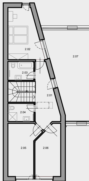
PŮDORYS 2.NP
