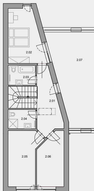
PŮDORYS 2.NP
