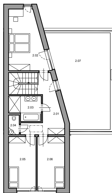
PŮDORYS 2.NP
