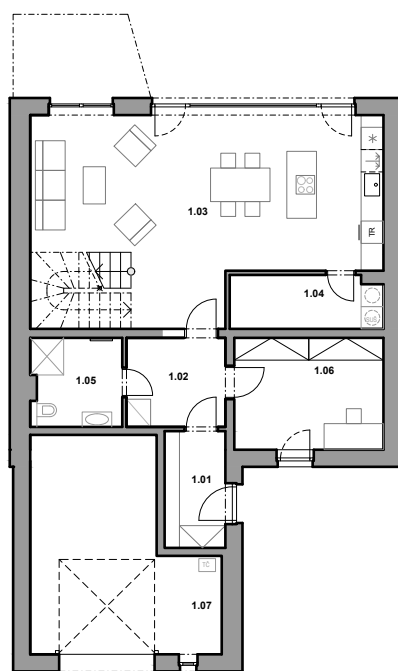
PŮDORYS 1.NP
